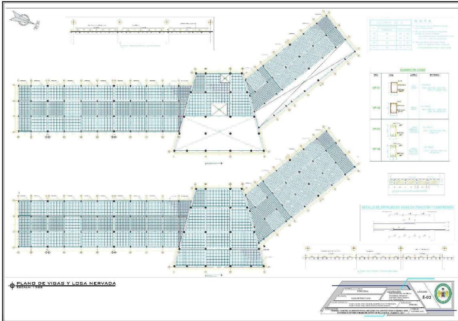
Figura 144 Plano de Aligerados (E-02)
