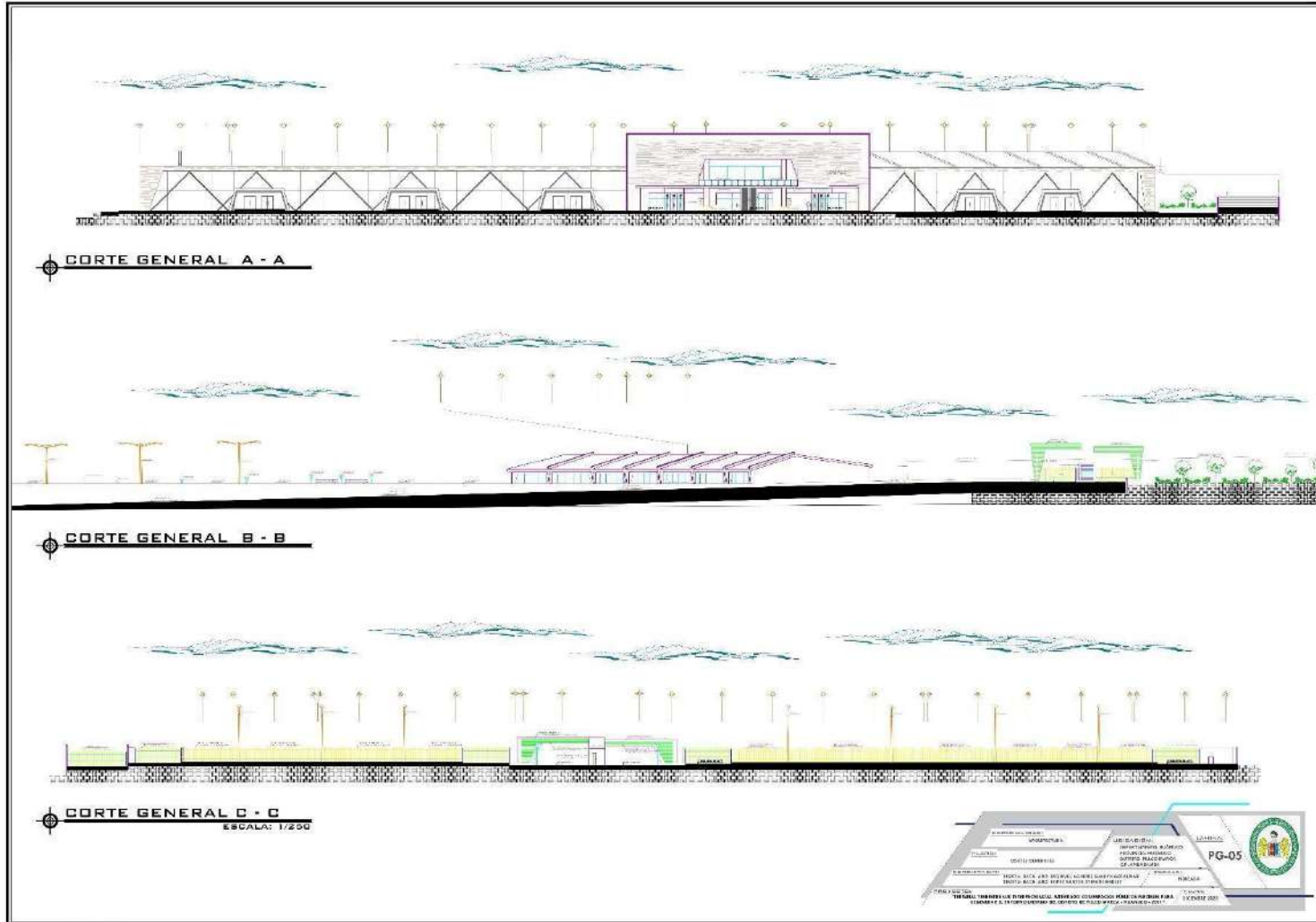
Figura 132 Plano de Cortes Generales (PG-05)
