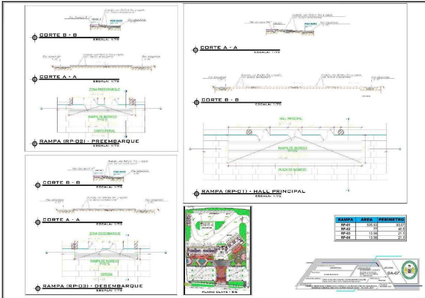
Figura 141 Plano de Detalles – Rampas Secundarias (DA-07)
