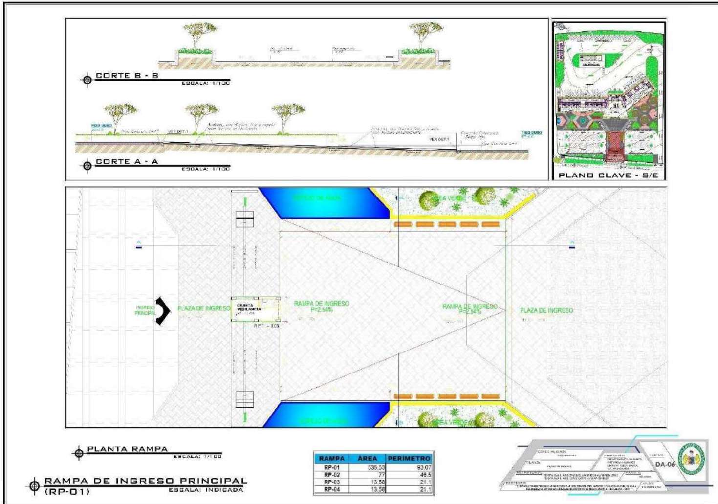
Figura 140 Plano de Detalles – Rampa Ingreso Principal (DA-06)
