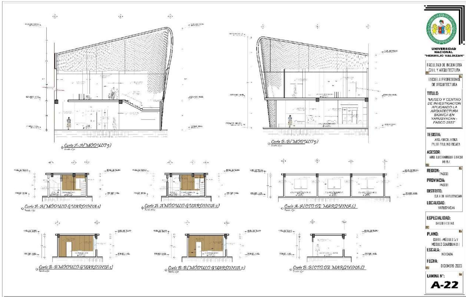
Cortes General del Módulo V y Complementarios
