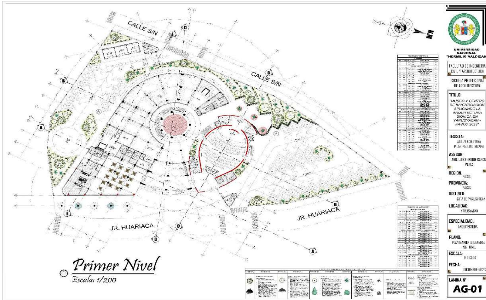
Planta General Primer Nivel
