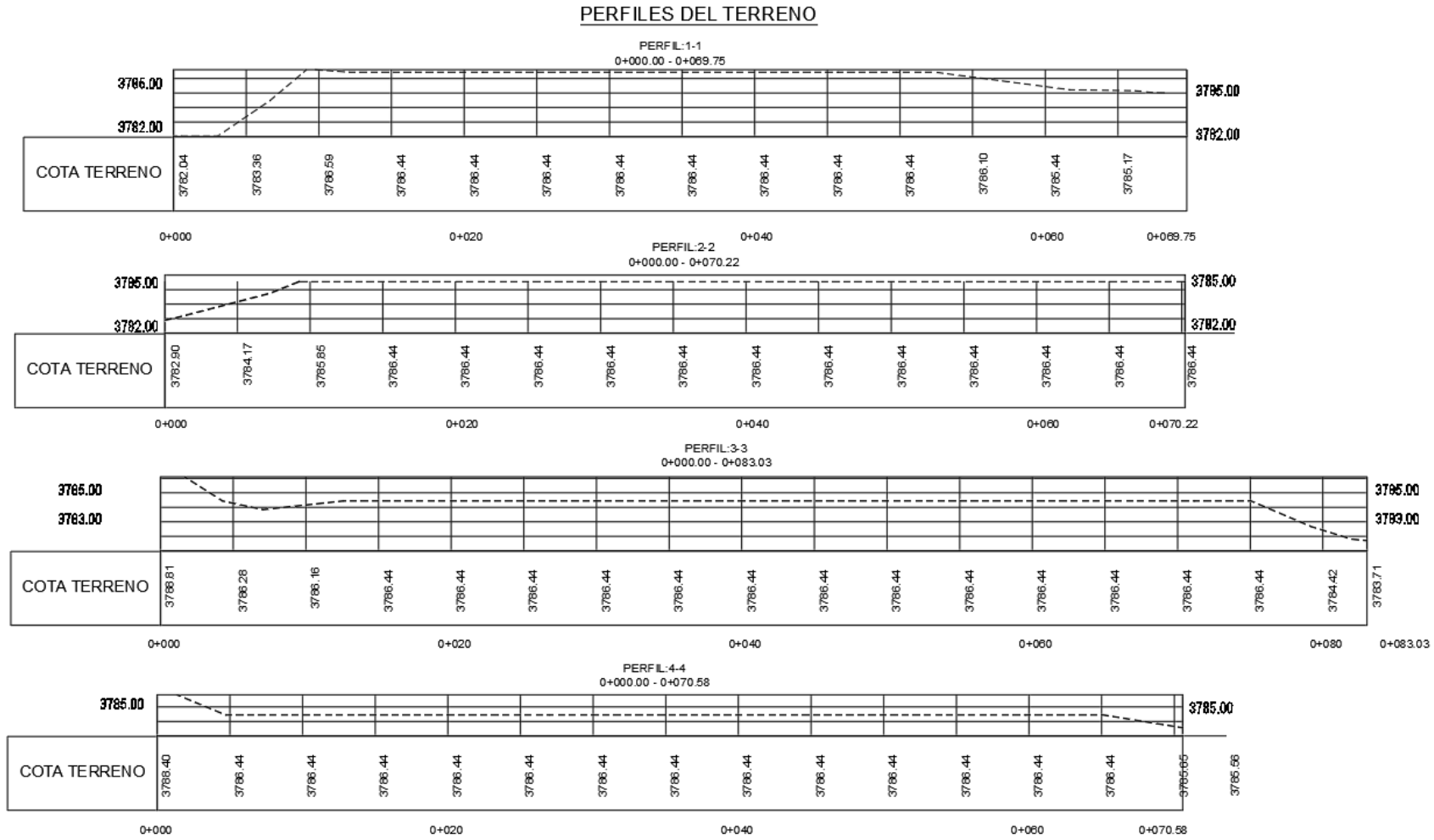
Figura N°35 Perfiles del terreno del proyecto
