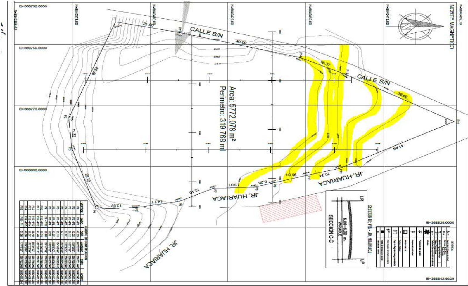
Figura N°36 Curvas de nivel del Terreno del Proyecto.
