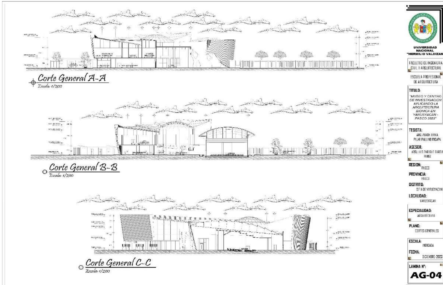
Cortes Generales I
