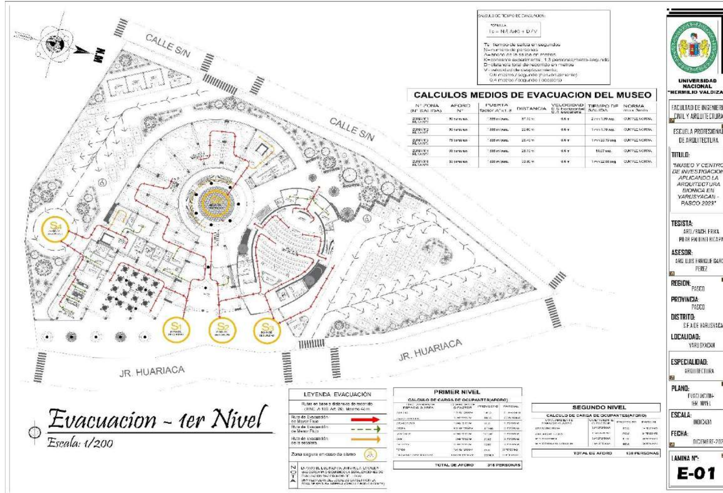
Plano de Evacuación del Primer Nivel
