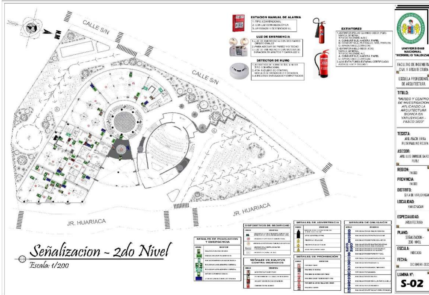
Plano de Evacuación del Segundo Nivel
