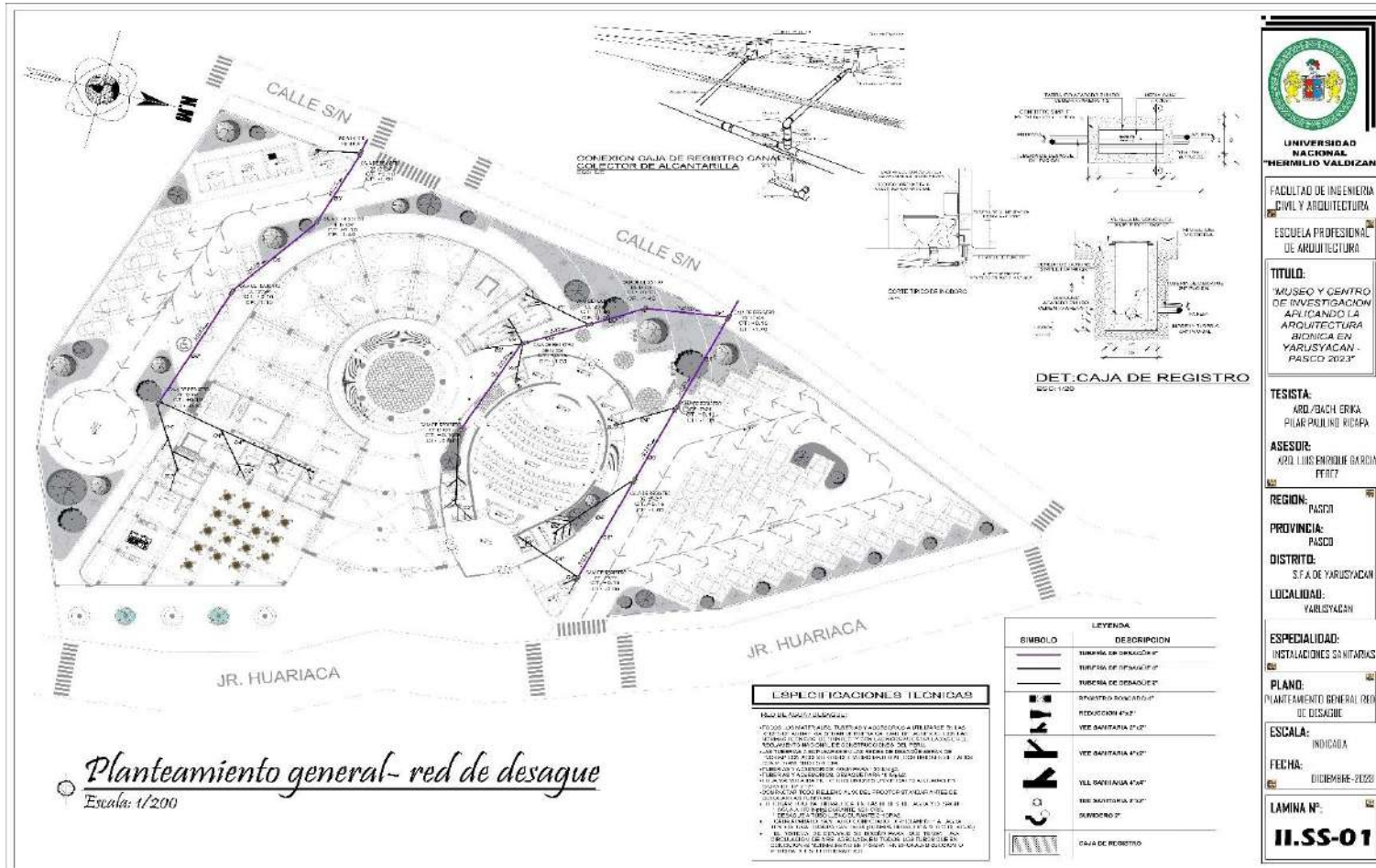
Plano General de Instalaciones Sanitarias - Desagüe
