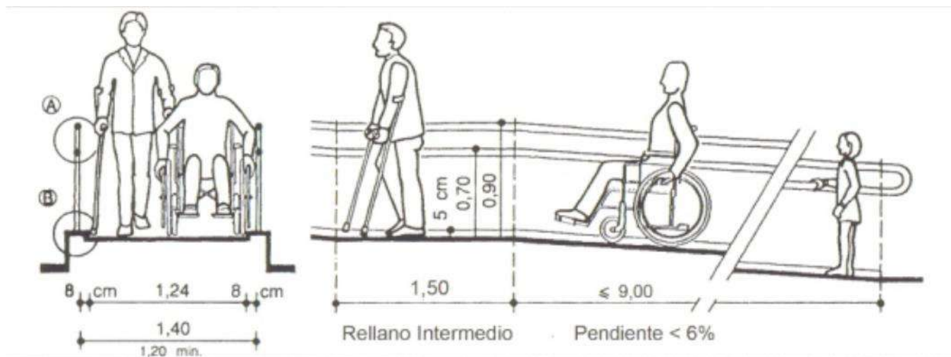
Dimensiones básicas de una rampa
