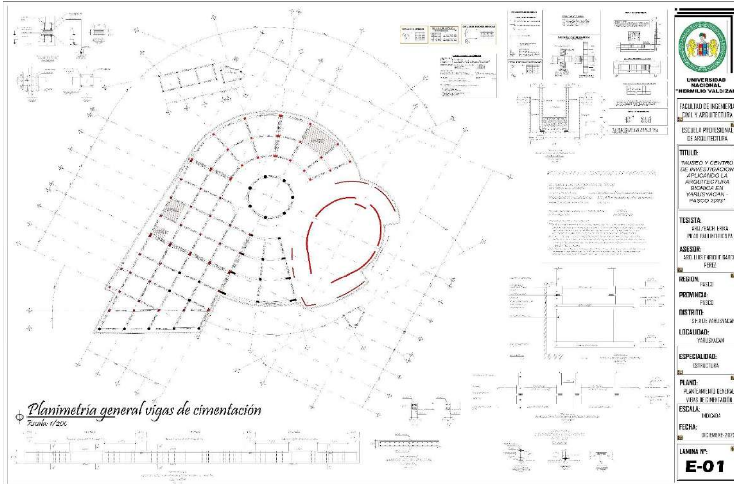
Plano General de Estructuras
