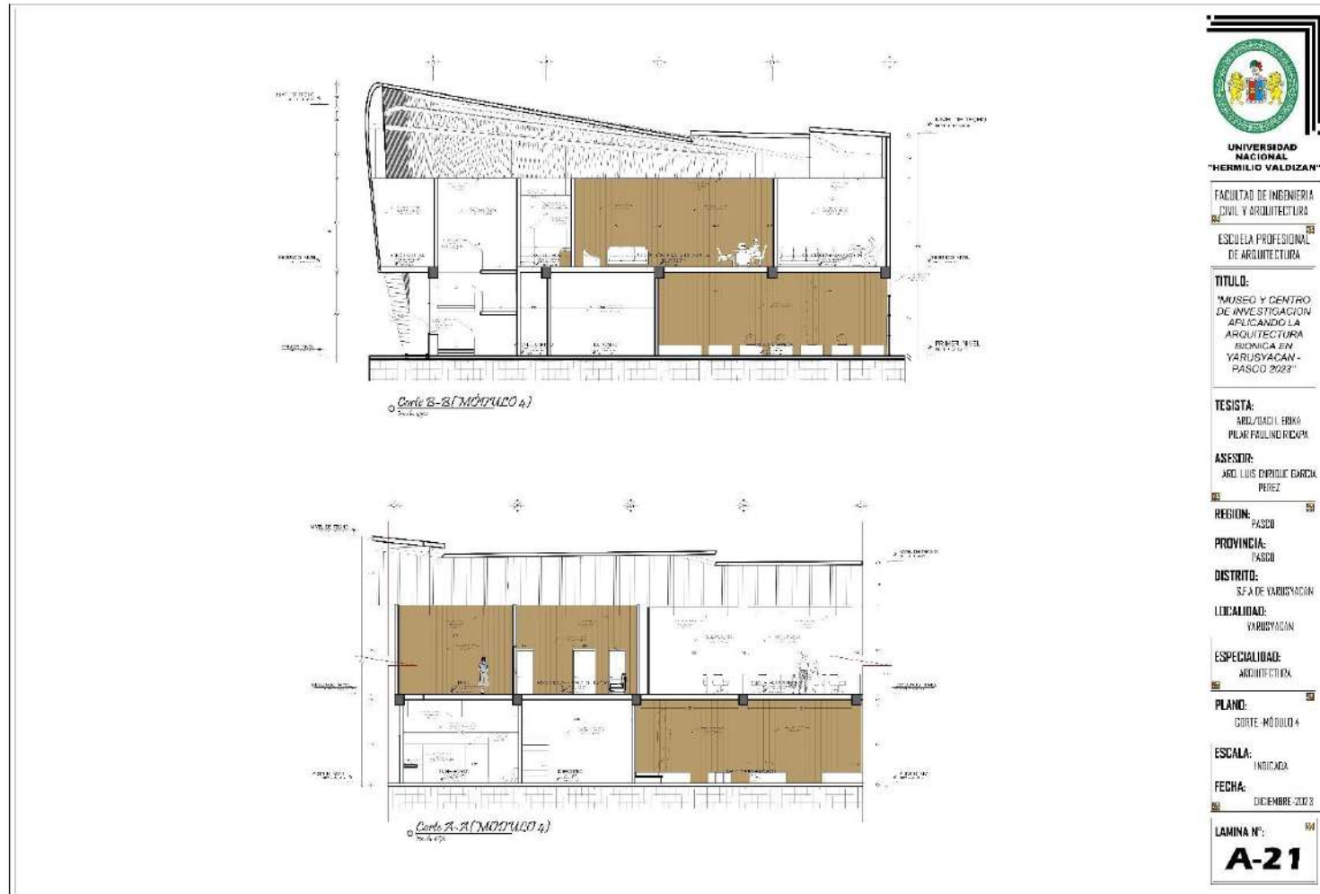
Cortes General del Módulo IV
