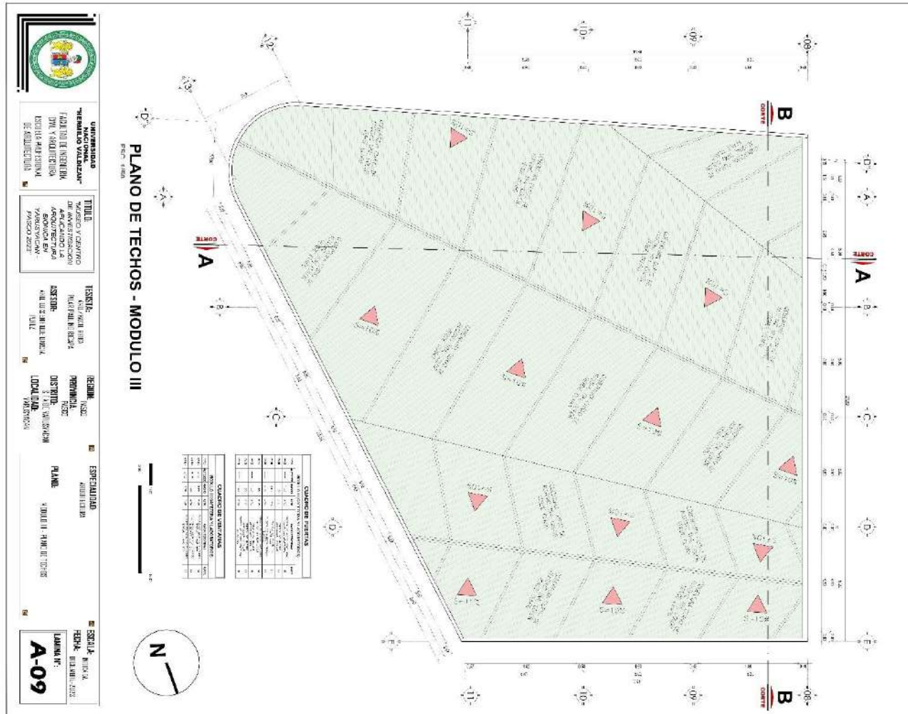
Plano de techos del Módulo III
