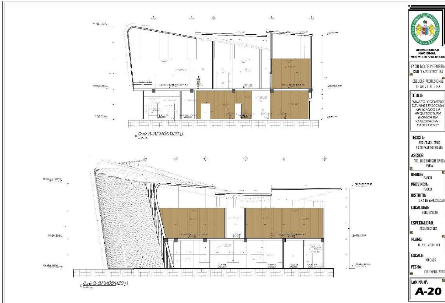
Cortes General del Módulo III
