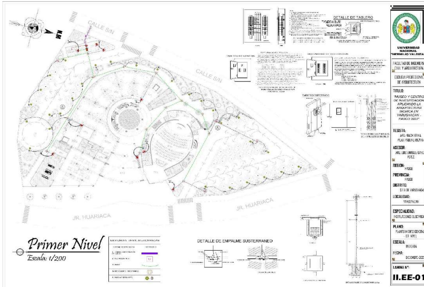
Plano General de Instalaciones Eléctricas
