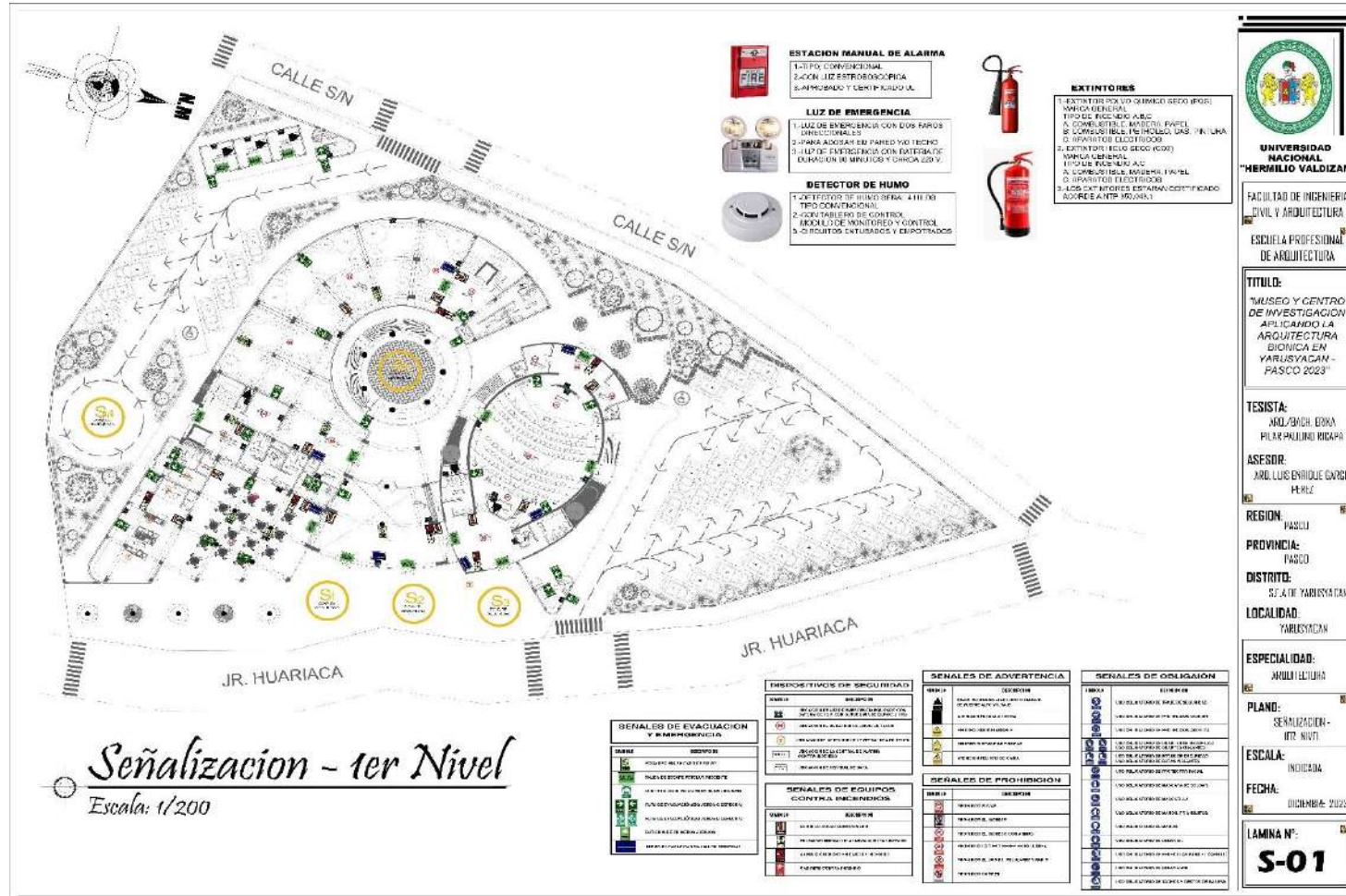
Plano de Señalización del Primer Nivel
